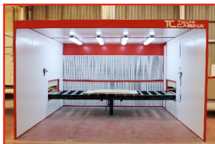
Fase 2: Cabina de pintura filtración vía seca dotada de gálipos y transportador de piezas
